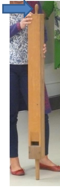
gedackte Orgelpfeife
